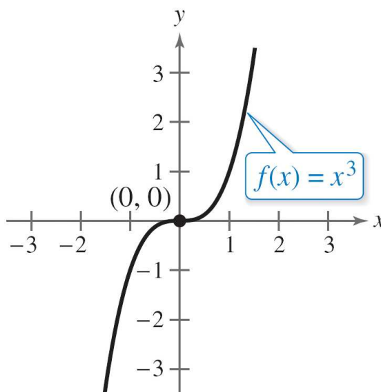
Cubic function
